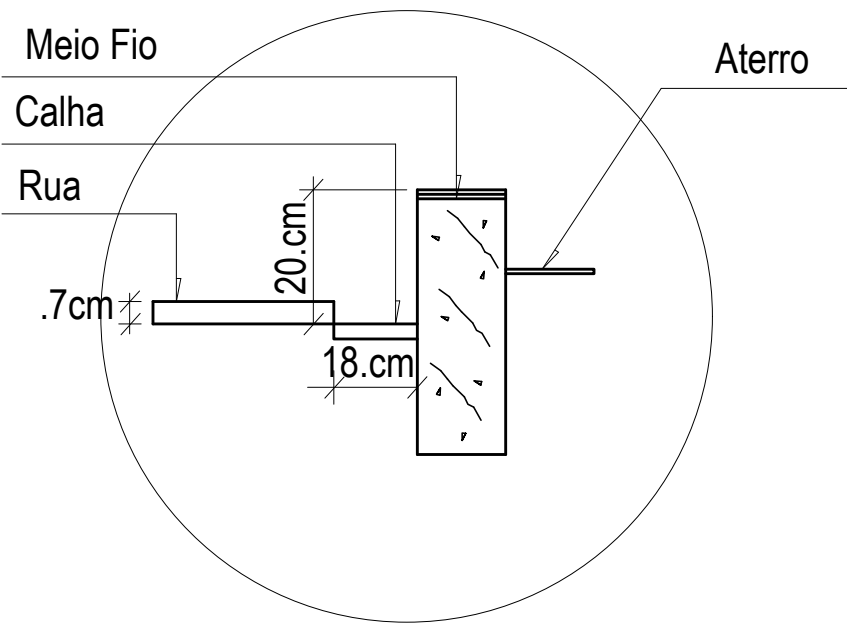
DETALHE DAS SARJETAS
